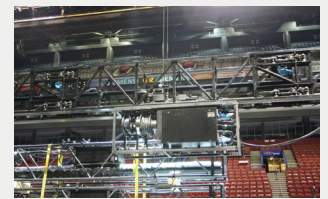
Un rail acrobatique avec chariot
